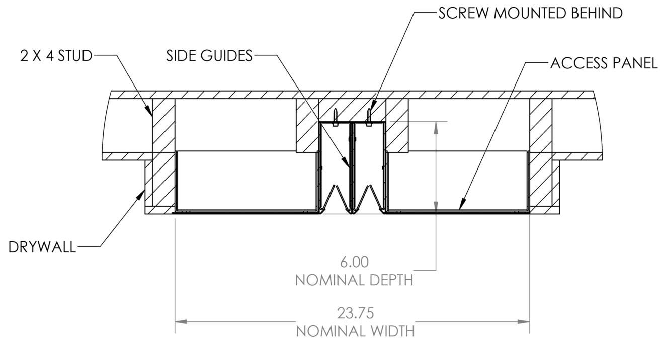
DOUBLE STUD WALL MOUNT
